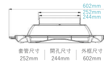
《DF-211A 四方吹》800CFM送風機雙出風口+Accubalance測試儀
