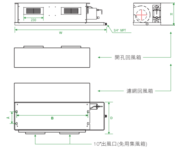
吊隱式送風機系列《負壓》規格表
