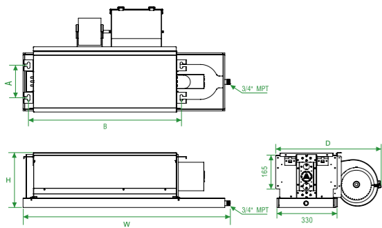
吊隱式送風機系列《正壓》規格表
